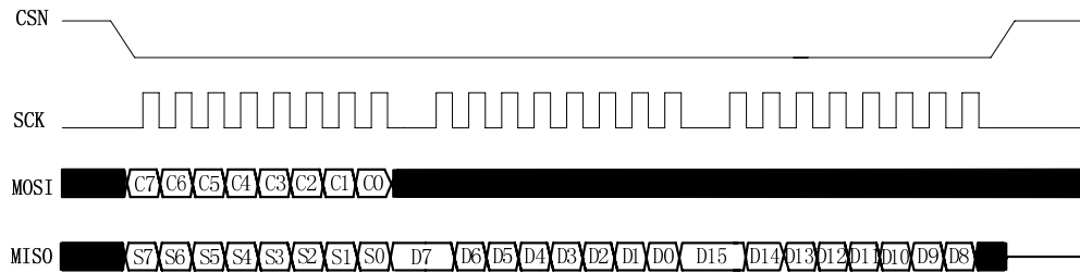
图7 SPI读操作
