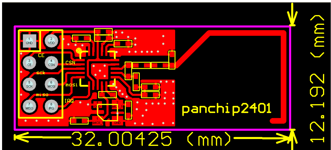
图12 顶层布线
