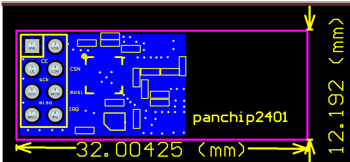
图13 底层布线
