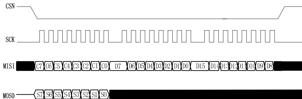
图8 SPI写操作
