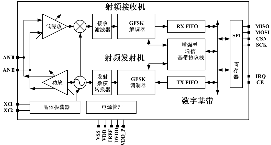
图1 XN297系统结构方框图
