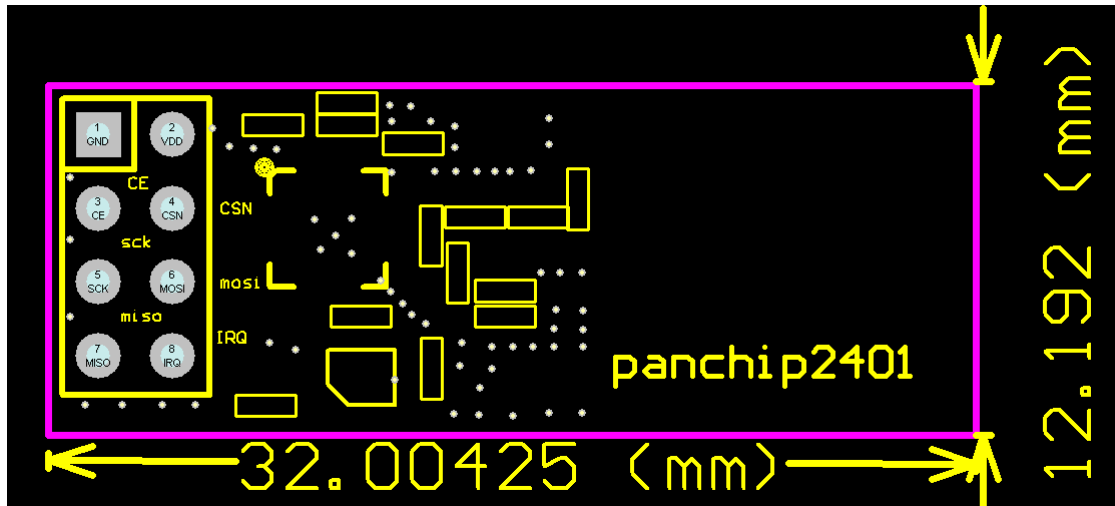
图11 顶层丝印
